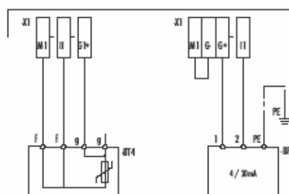
Sonda Riello
